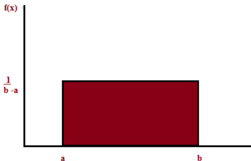
Figura 67. Distribución uniforme
