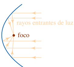
FIGURA 10.1.20 Superficie reflectora parabólica
