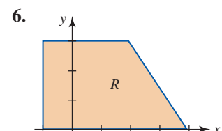
FIGURA 14.1.11 Región de integración del problema 6
