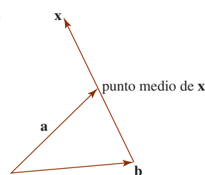
FIGURA 11.1.16 Vectores del problema 38
