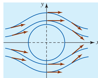
FIGURA 15.7.6 Campo de velocidades del problema 40
