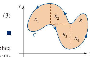
FIGURA 15.4.3 Región R descompuesta en cuatro subregiones
