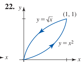
FIGURA 15.1.12 Curva del problema 22
