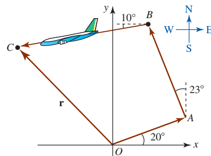
FIGURA 11.1.23 Vectores del problema 50
