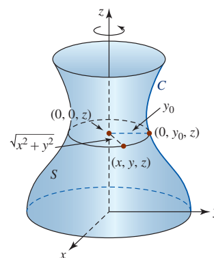
FIGURA 11.8.9 Superficie S de revolución
