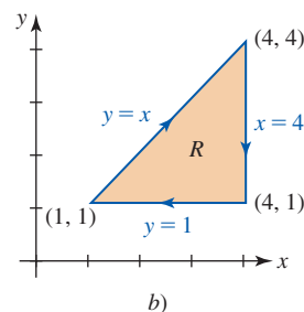
FIGURA 14.9.2 La imagen de S es R
