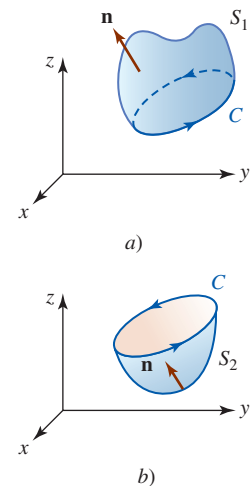
FIGURA 15.8.6 Dos superficies con la misma frontera C
