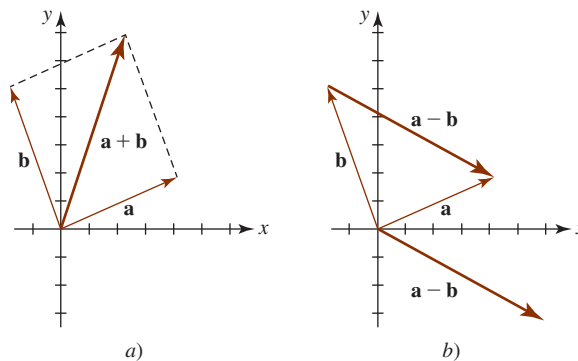
FIGURA 11.1.12 Gráficas de los vectores del ejemplo 5
