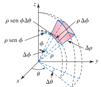
FIGURA 14.8.7 Cuña esférica
