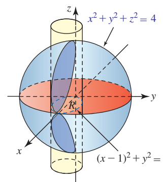
FIGURA 14.6.3 Superficie del ejemplo 2
