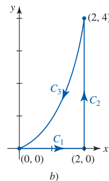
FIGURA 15.1.6 Curva C en el ejemplo 3
