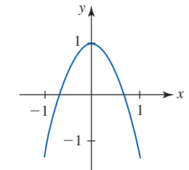
a) y = 1 - 2x^2 , -\infty < x < \infty
