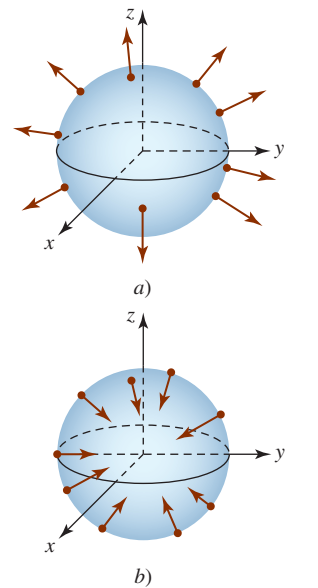
FIGURA 15.6.7 Orientación hacia fuera en a); orientación hacia dentro en b) en el ejemplo 4
