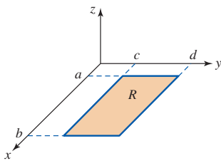
FIGURA 14.2.4 La región rectangular es tanto del tipo I como del tipo II
