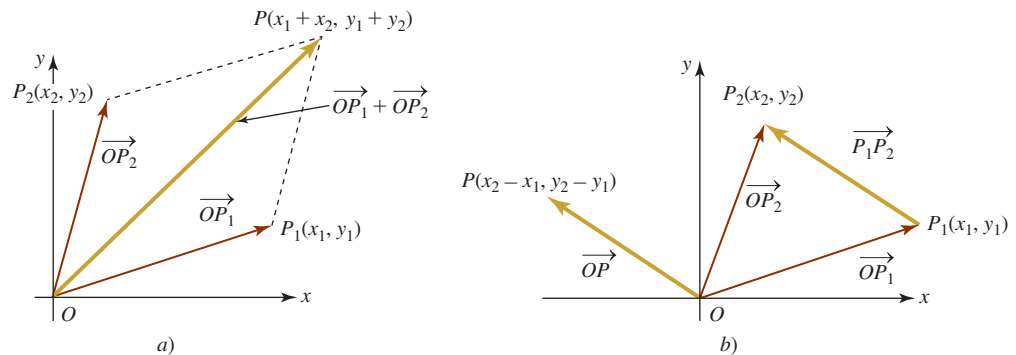
FIGURA 11.1.9 Resta de vectores
