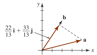
FIGURA 11.3.6 Proyección de a sobre b
