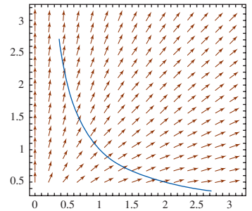
FIGURA 15.2.5 Curva y campo vectorial del ejemplo 2
