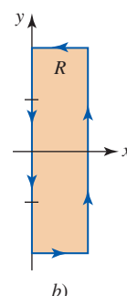
FIGURA 15.8.2 Superficie del ejemplo 1
