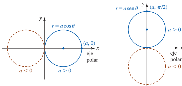
a) Centros sobre el eje x b) Centros sobre el eje y FIGURA 10.5.12 Círculos que pasan por el origen con centros sobre el eje
