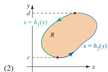
b) R como una región tipo II
