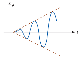
FIGURA 16.4.11 Resonancia pura
