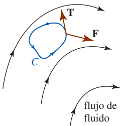
FIGURA 15.2.9 Curva cerrada en un campo de velocidades
