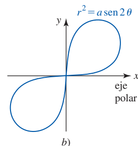
b) FIGURA 10.5.13 Lemniscatas
