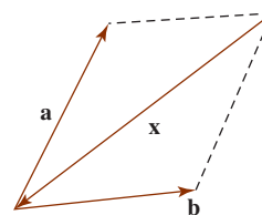
FIGURA 11.1.15 Vectores del problema 37
