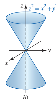
FIGURA 11.8.10 Cono de un solo manto a); cono de doble manto en b)
