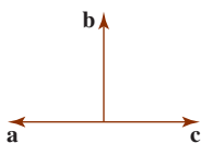
FIGURA 11.1.14 Vectores del problema 36
