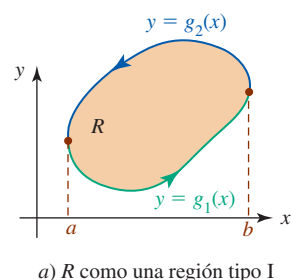
a) R como una región tipo I
