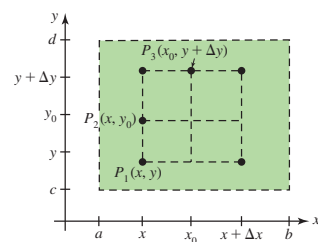
FIGURA 13.4.2 Región rectangular en el teorema 13.4.1
