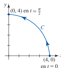
FIGURA 15.1.4 Curva C del ejemplo 1
