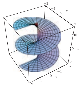
FIGURA 15.6.4 Helicoides del ejemplo 3
