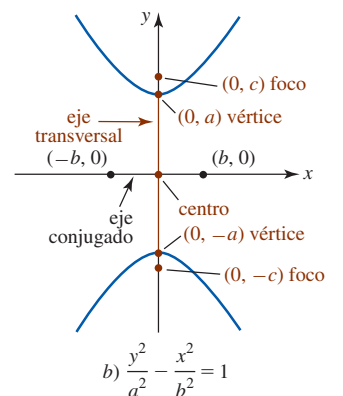
FIGURA 10.1.14 Resumen gráfico de las ecuaciones (17) y (18)
