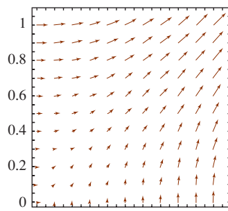
FIGURA 15.2.11 Campo vectorial conservativo del ejemplo 5
